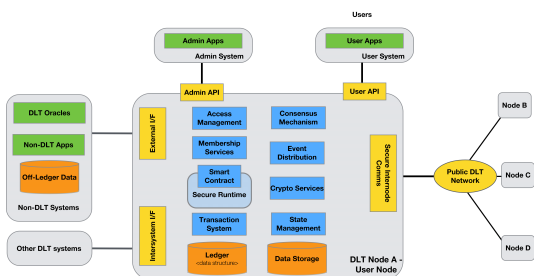
[그림 2] TR 3242에서 사용한 참조아키텍처의 시스템 뷰
