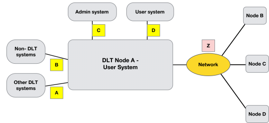
(그림 3) TR 3242에서 사용한 데이터 흐름
